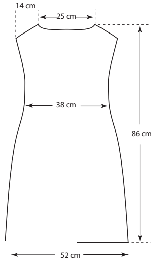
Predný/zadný diel
